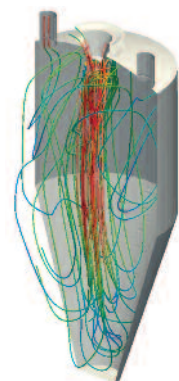
Simulação CFD (Comput. Fluid Dynamics)
